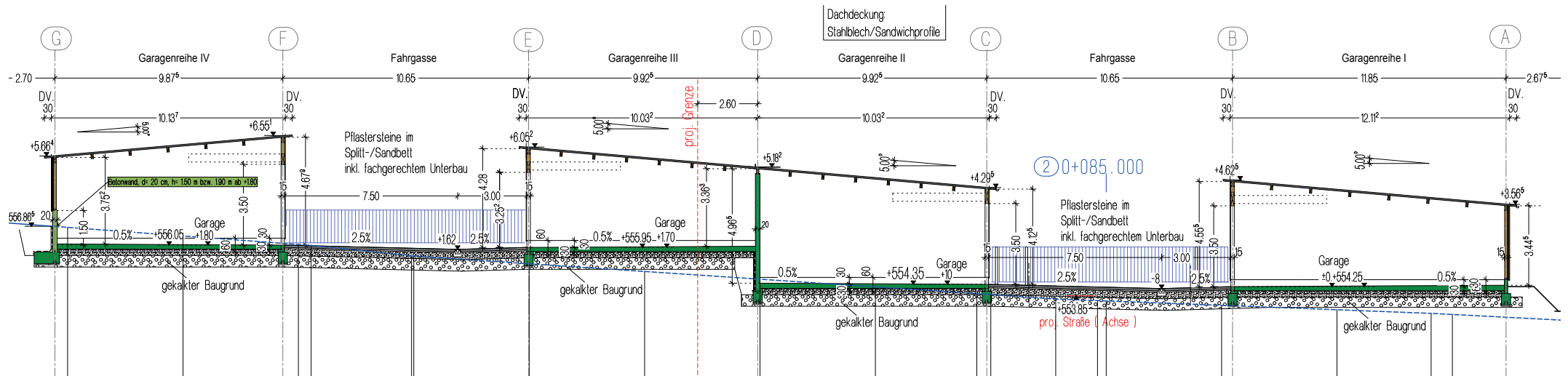
Schnitt mit Höhenübersicht.
